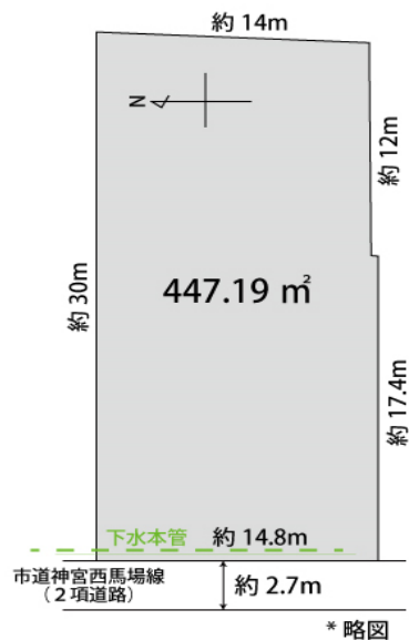
敷地図
